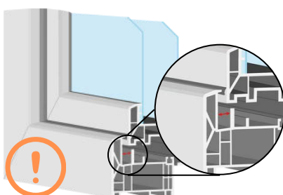
Mitteldichtung: Abstand min. 12 mm
