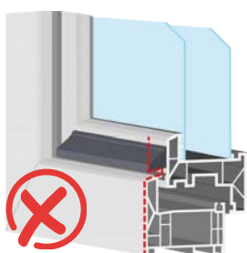
Flächenversetztes Fenster mit Wetterschenkel
